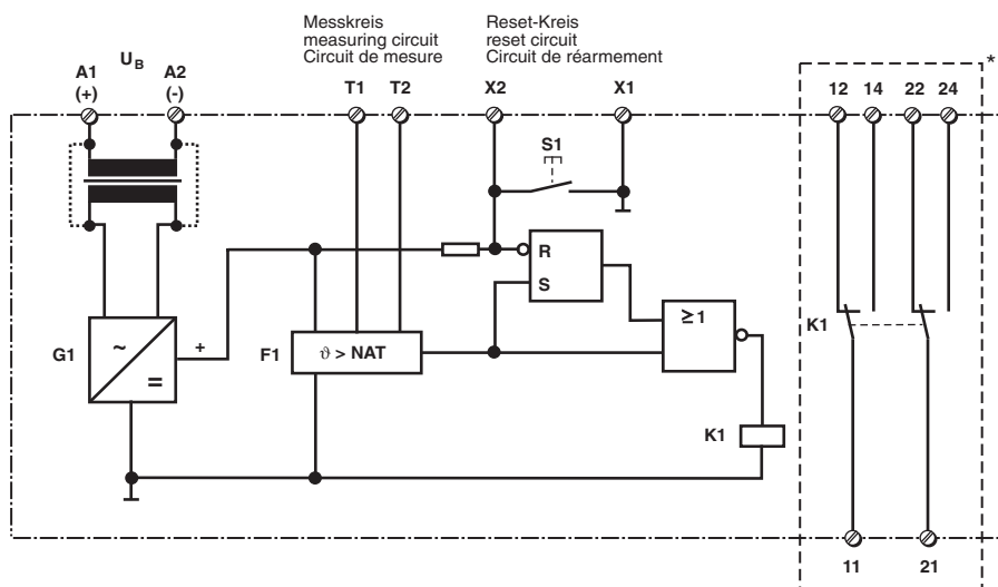
Fig. 1: Schematisches Schaltbild
