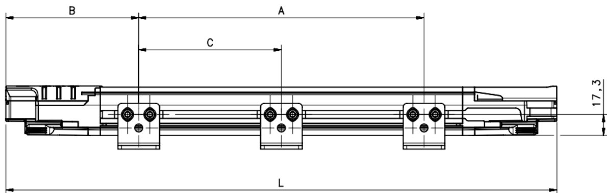
Fig. 19 – Light curtain dimensions
