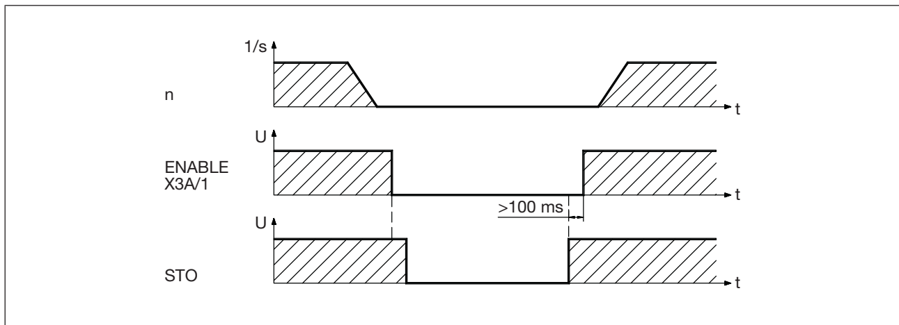
Fig.: Safety function STO
