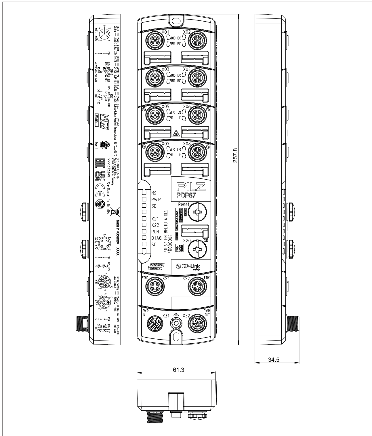
Fig.: Dimensions
