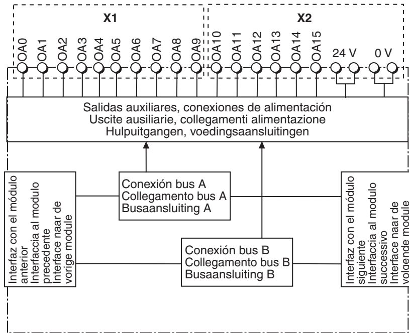
Fig. 1: Schema connessioni
